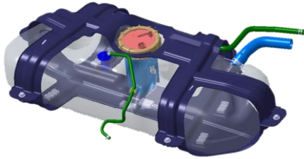
高圧密閉樹脂製燃料タンク
